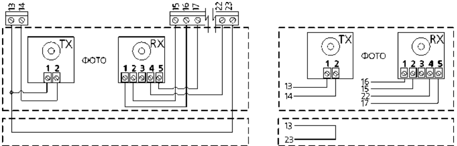
Рисунок 3В. Схема подключения только одного фотоэлемента Photo
